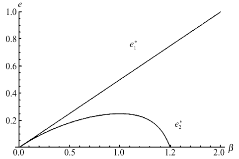
图 1 0 < k \leq k_0 时 e 和 \beta 的关系: c = 0.5, k = 3
